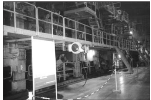
2. kép. Papírgép
